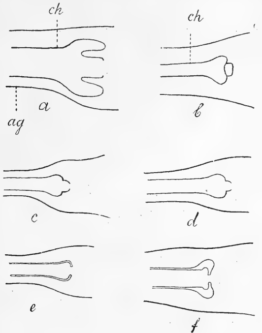
Рис. 1. Начальная часть выводного отдѣла ядовитой железы: а— Parabuthus planicauda Poc. б— Buthus eupeus (C. L. Koch), с— Hemiscorpion lepturus Peters, д— Euscorpium carpathicus (L.), е— Pandinus peeli Poc. (juv.) ф— Teuthraustes witti (KrpIn).
