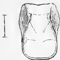
Рис. 3. Amuria brunneri , sp. n. ♂. Pronotum.
