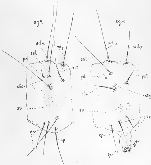
Рис. 2. — Второй (sg. 2) и четвертый (sg. 4) абдоминальные сегменты гусеницы Hepialus lutuli L и п., первой фазы, сбоку, при большемъ чѣмъ на рис. 1 увеличеніи. Setae: sd. a — subdorsalis anterior, sd. p — subdorsalis posterior, sst — suprastigmatalis, pd — praedorsalis (но, можетъ быть, вторая suprastigmatalis), pst — poststigmatalis, sbs — substigmatalis, ep — три extrapodales, ip — intrapodalis, sv — отсутствующая supraventralis (пунктиръ, указующій ея мѣсто, слишкомъ коротокъ и долженъ быть удлиненъ значительно въ сторону носсегментальнаго края сегмента); stg — stigma; передній и задній края сегментовъ, равно какъ и поле подъ tuberculum substigmatale, усыяны мельчайшими spinulae. Zeiss, obj. D, oc. 1.
