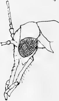
Рис. 9. Boreus chadzhi-gireji , sp. n. ♀. Голова сбоку.
