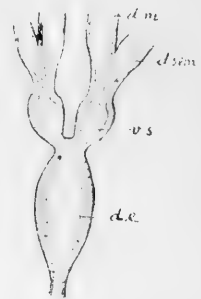
Рис. 2. Melampsalta tibialis Pa p z. Схема конечнаго отрѣзка мужскаго полового аппарата. d. sem.—сѣменной каналецъ, de ductus-ejaculatorius, d. m. придаточныя железы, v. s.—vesicula seminalia.
