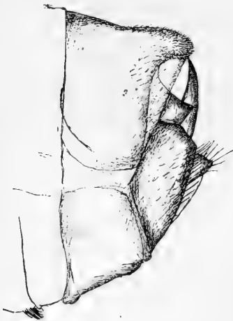
Рис. 10. Anisogamus flavipunctatus , sp. n. ♂. Конец брюшка сбоку.
