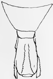
Рис. 7. Boreus navasi , sp. n. ♀. Конецъ брюшка сверху.
