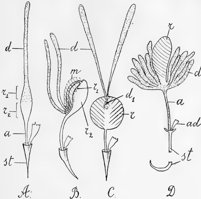
Рис. 2. Схемы ядовитыхъ аппаратовъ: Megachile (A), Scolia (B), Vespa (C) и Vipio (D). Пунктированные части органовъ соответвуютъ отдѣламъ, въ стѣнкахъ которыхъ сосредоточены железистыя клѣтки.
