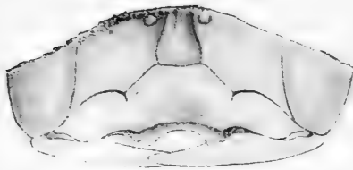
Рис. 1. Cerceris ansa , sp. n. ♀. Clypeus.
