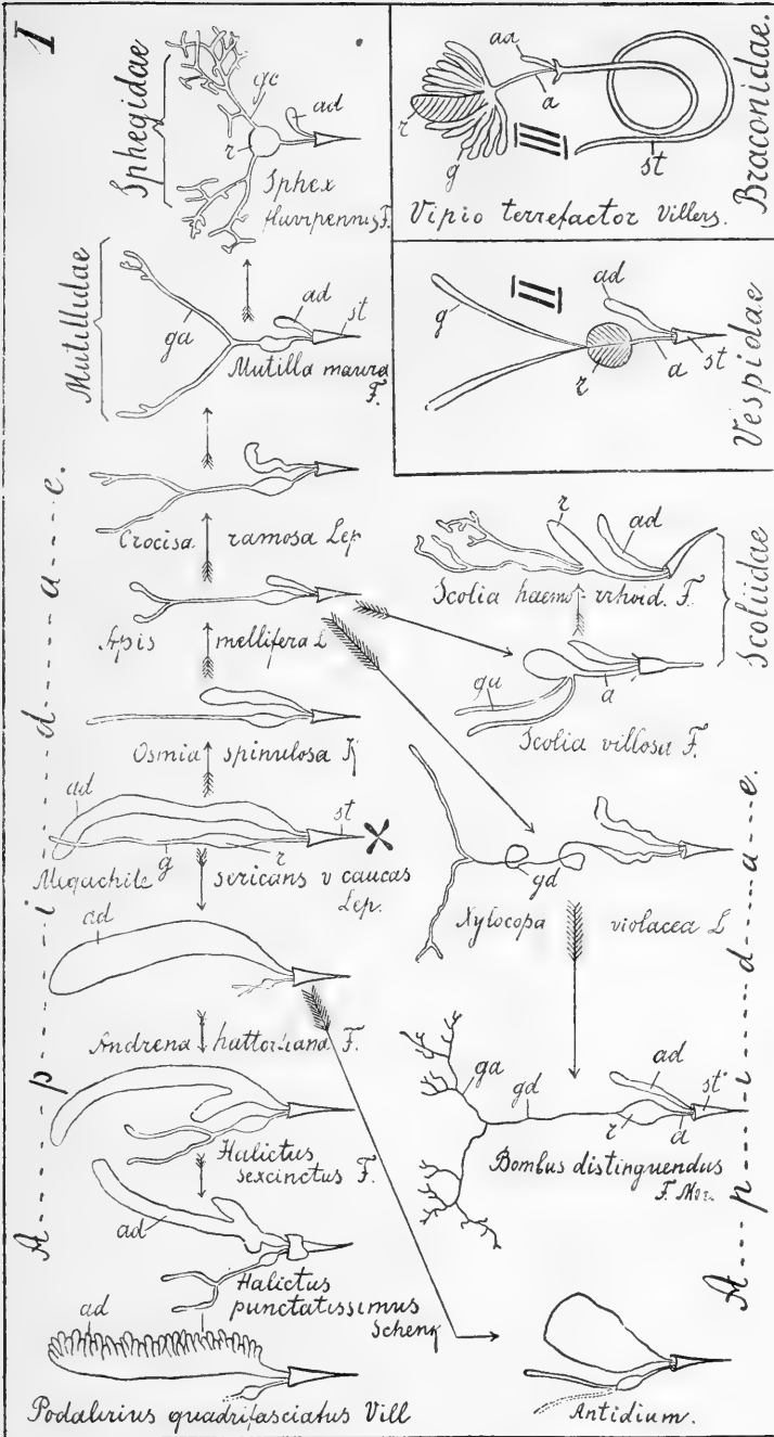
Рис. 1. Наружная морфология ядовитых аппаратов Нумерптера (схема). I — тип Apiidae (у семейств: Apiidae , Sphegidae , Scoliidae и Mutillidae ); исходной формой принимается Megachile sericans var. caucasica L. p. (X); по ходу стрелок расположены ядовитые аппараты, постепенно уклоняющиеся в ту или иную сторону в степени развития своих частей. II — тип Vespididae . III — тип Braconidae . a — выводящий канал резервуара кислотной железы; ad — щелочная железа; g — кислая железа (не втягивающаяся); ga — головная ветви кислотной железы; gc — парная втягивающаяся трубка кислотной железы; gd — непарная часть кислотной железы; r — резервуар; st — жало.
