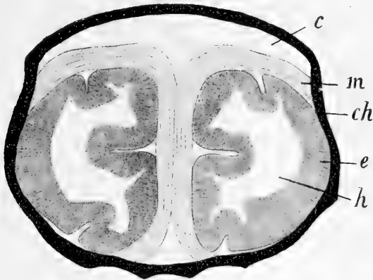
Рис. 2. Urodacus manicatus Thos. Поперечный разрѣзъ постъанального сегмента (съ ядовитыми железами дефинитивнаго типа). с — полость сегмента; ch — хитинъ кожныхъ покрововъ; е — эпителиальная стѣнка ядовитой железы, образующая складки, направленныя въ полость органа; h — полость ядовитой железы; m — поперечнополосатая мускульная оболочка железы.
