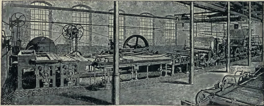
6. ábra. A síkszítás papirosmerítő-gép távlati képe.
