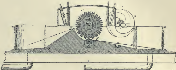
2. ábra. A nagyoló-foszlató hosszanti metszete.
