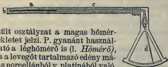
2. ábra. Petersen fémpirométere.
