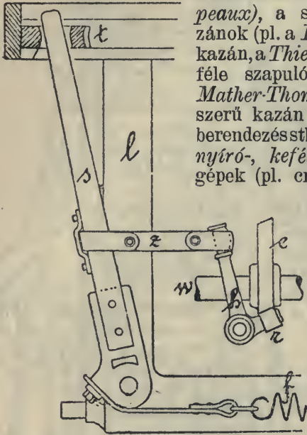
4. ábra. Vetőszerkezet alsó ostonnal.
