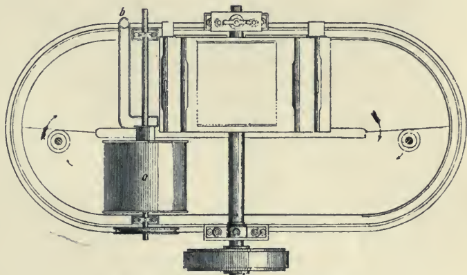
3. ábra. A nagyoló-foszlató alaprajza.
