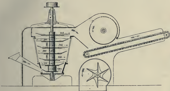
1. ábra. Chrigh-ton-féle csomóbontó.
