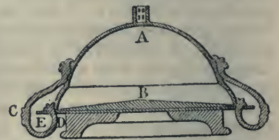
3. ábra. Nagyobb csésze berakása. A csésze B porcellánbiscuitlemezre van fordítva, mely D chamotte-lemezen fekszik.
