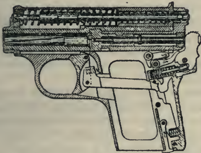
4. ábra. Frommer-Baby pisztoly metszetben.
