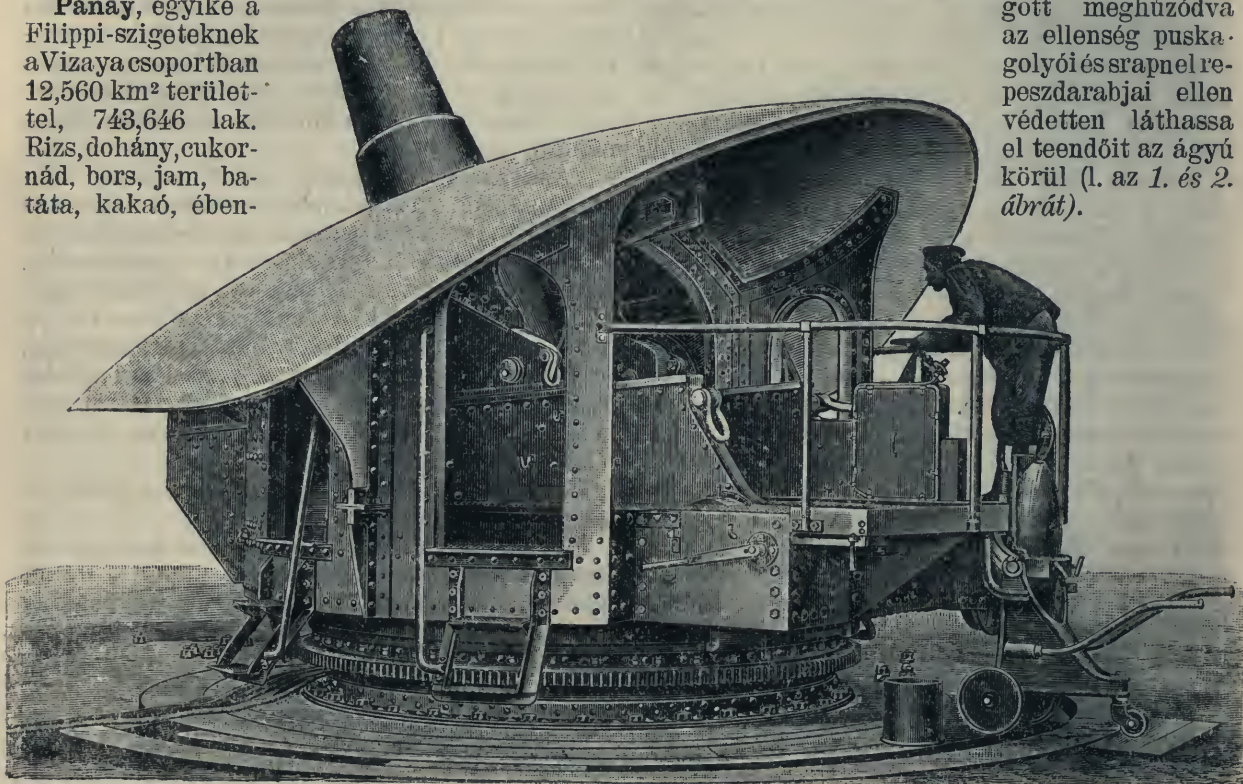
1. ábra. 28 cm. Krupp-féle tarack tengerparti lövegtalpban védőpajzs-szal.
