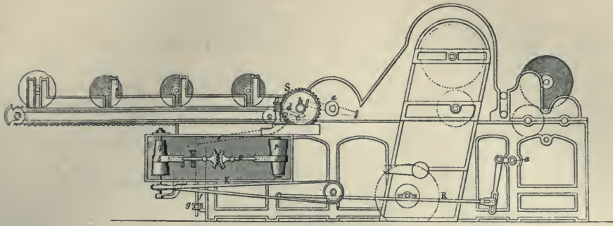
2. ábra. Léces verőgép (Batteur).
