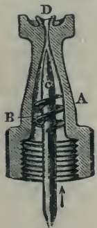
1. ábra. Körting-féle szórós porlasztó.
