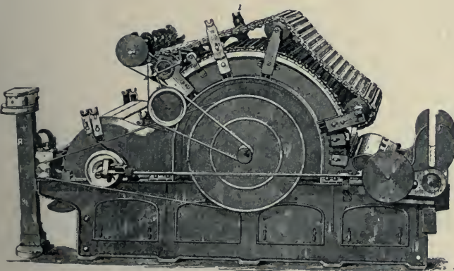
4. ábra. Fedeles kártológép mozgó lécekkel.
