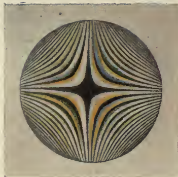
3. Két, a tengellyel párhuzamosan metszett lemez keresztezve: hiperbolák.
