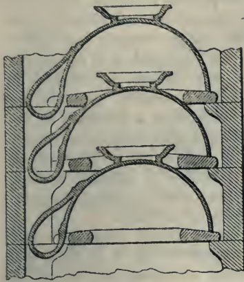
4. ábra. Csészék berakása.
