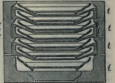
1. ábra. Tányérok berakása. t t a tokok.
