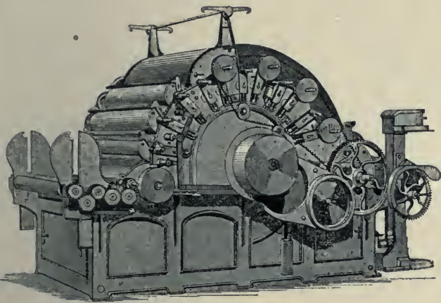
3. ábra. Hengeres kártológép.
