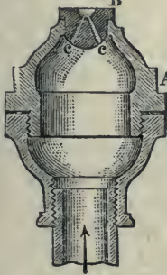
2. ábra. Kétsugarú por- lasztó.
