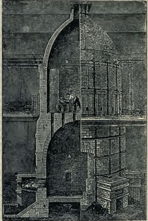
6. ábra. Porcellánégető kemence. A alsó kamra, B felső kamra, a a a a tüzhelyek.
