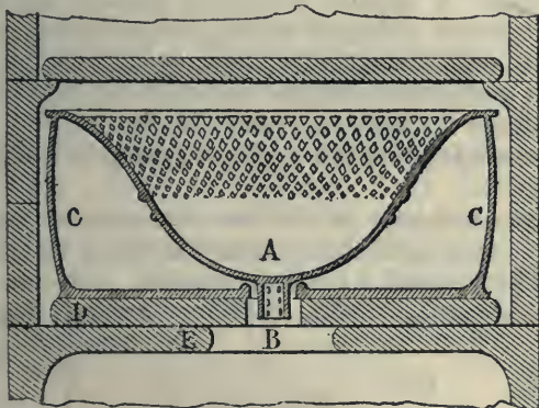
5. ábra. Könnyen elhúzódó csészének támasszal való berakása. A a porcellántárgy, mely a C porcellánbiscuitből készített támaszon nyugszik. D és E a tok.
