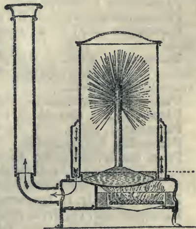
A Ventzki-rendszerű pároló készülék vázlatos hosszmetzete.
