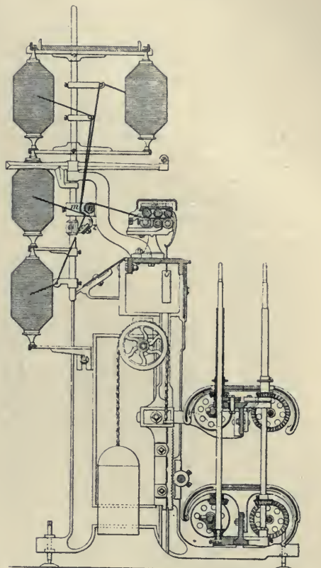
6. ábra. Fleyer-rendszerű előfonógép.
