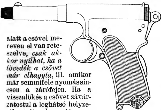
3. ábra. Frommer-pisztoly nézetben.
