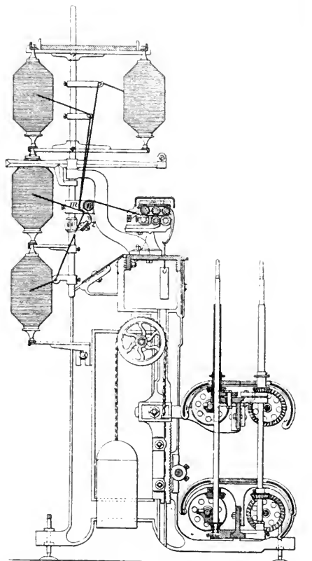
6. ábra. Fleyer-rendszerű előfonógép.
