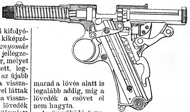
2. ábra. Frommer-pisztoly metszetben.
