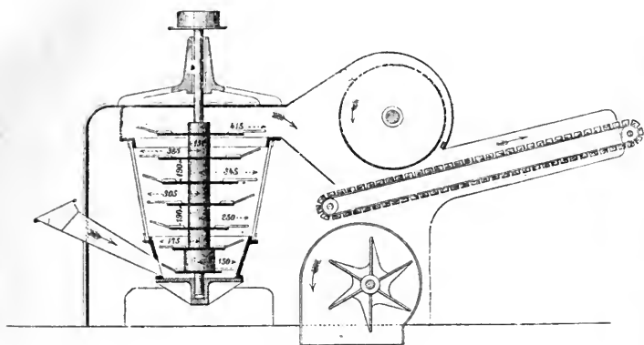
1. ábra. Chrington-féle csomóbontó.
