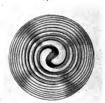
6. Cukor: nem teljesen kör alakú gyűrűk.
