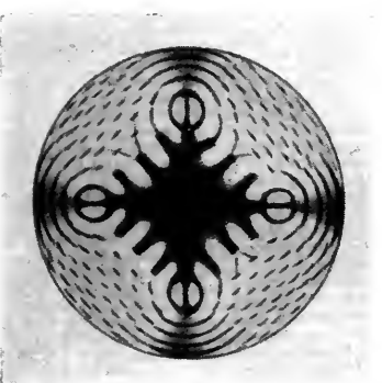
10. Arragonit keresztezve nátriumfényben.
