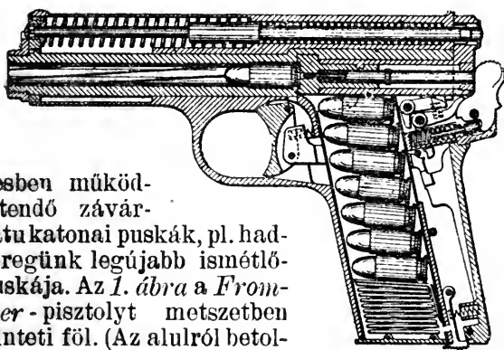
5. ábra. Frommer-Stop pisztoly met-szetben
