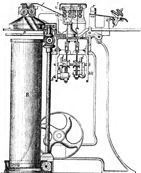
5. ábra. Nyújtógép (Laminoir).
