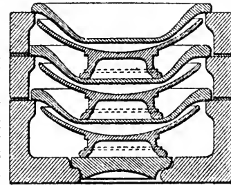
2. ábra. Tálak berakása.
