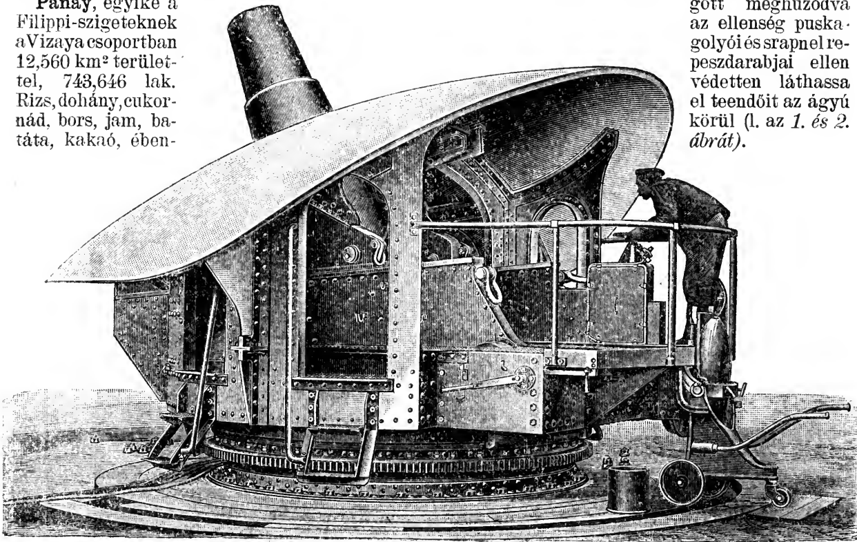
1. ábra. 28 cm. Krupp-féle tarack tengerparti lövegtalpban védőpajzs-szal.
