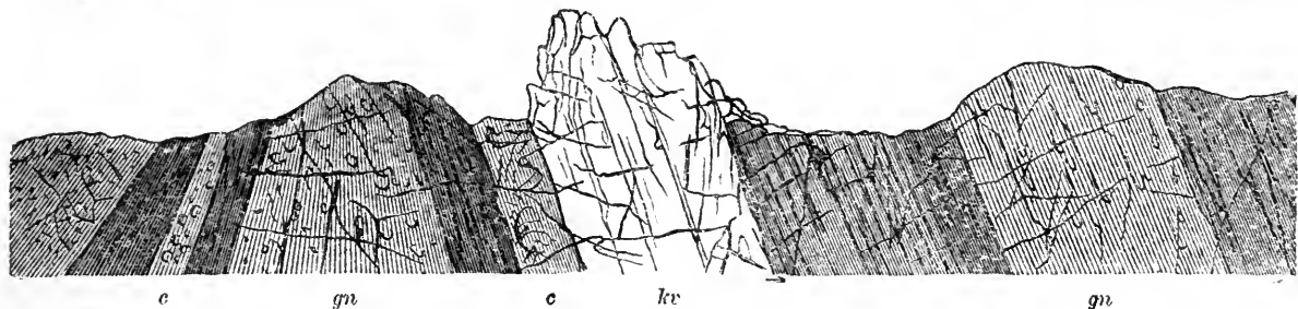
2. ábra. A kvarcittal (Pfahl) geológiai keresztmetszete. gn = különböző gnájstfélések, kv = kvarcit (Pfahl), c = hellefintaszertű kőzet.
