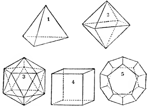
1. Tetraéder. 2. Oktaéder. 3. Ikozaéder. 4. Hexaéder. 5. Dodekaéder.
