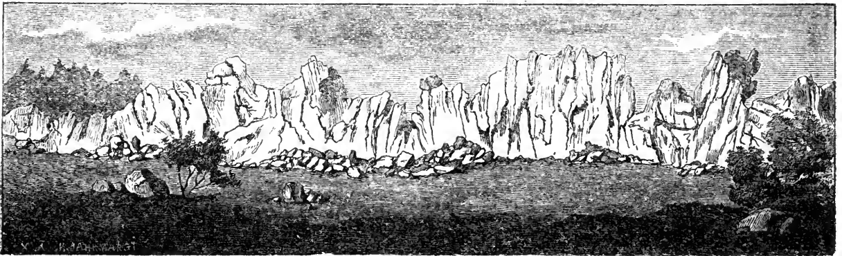
1. ábra. A kvarcittal (Pfahl) a cseh-bajor határhegységben.
