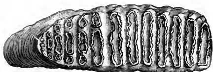
6. Az Elephas antiquus zápfoga. \frac{1}{6} .
