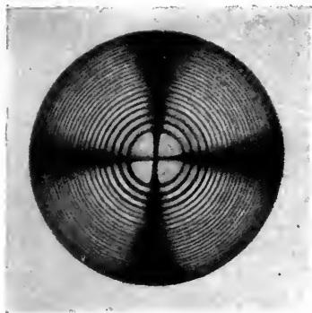
1. Mézspát: fekete kereszt.
