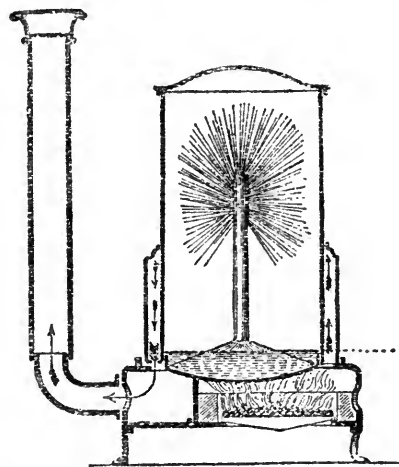
A Ventzki-rendszerű pároló készülék vázlatos hosszmetsete.
