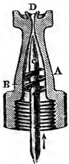
1. ábra. Körting-féle srófos porlasztó.
