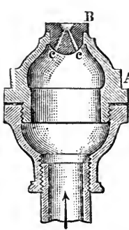
2. ábra. Kétsugarú por- lasztó.
