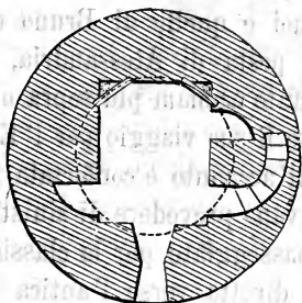
PIANTA DEL NURAGHE NORBELLO
