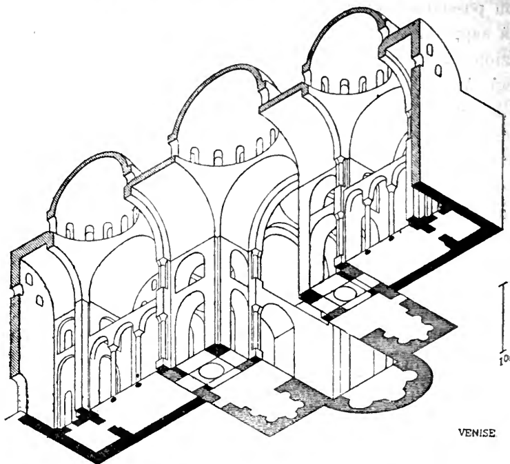
Pianta e spaccato trasversale di S. Marco a Venezia
