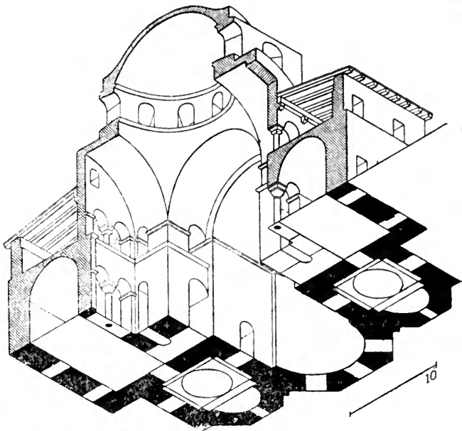
Pianta e spaccato di S. Sofia in Salonicco.
