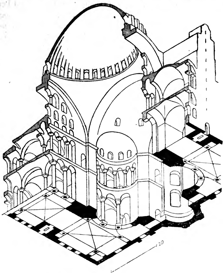
Pianta e spaccato di S. Sofia in Costantinopoli.
