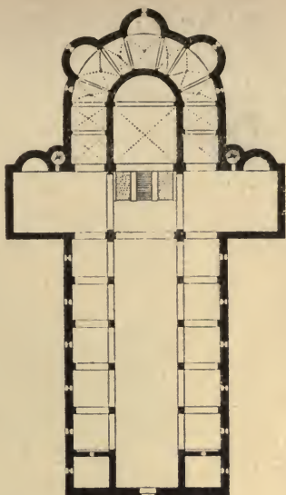
Duomo d'Acerenza: 1 : 1000 1
