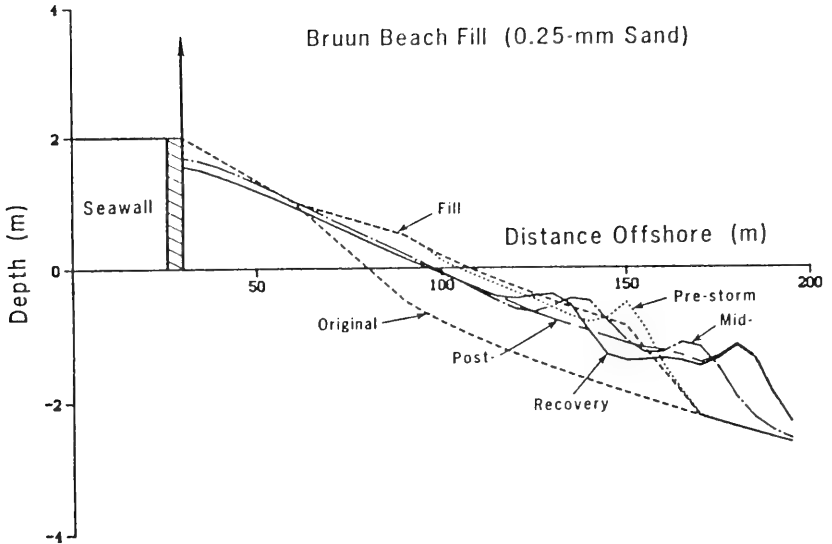
a. 0.25-mm beach
