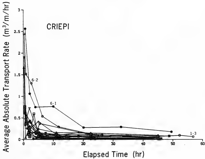
a. CE data, 16 cases
