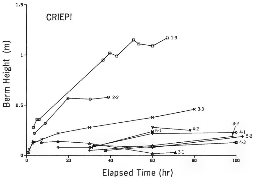
b. CRIEPI data
