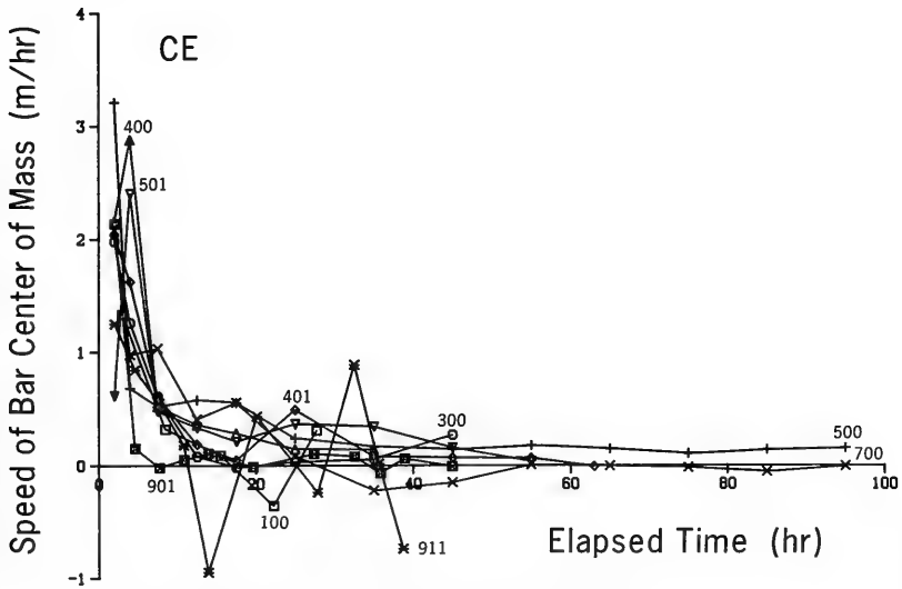
a. CE data, bar center of mass
