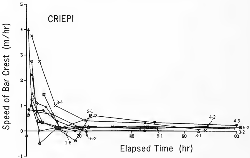
d. CRIEPI data, bar crest
