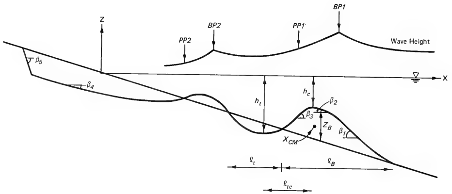
a. Bar profile
