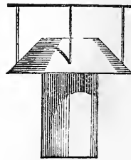
Ejecting Ventilator.
