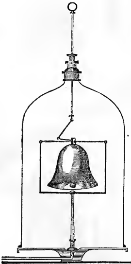
BELL IN VACUO. Fig. 82.
