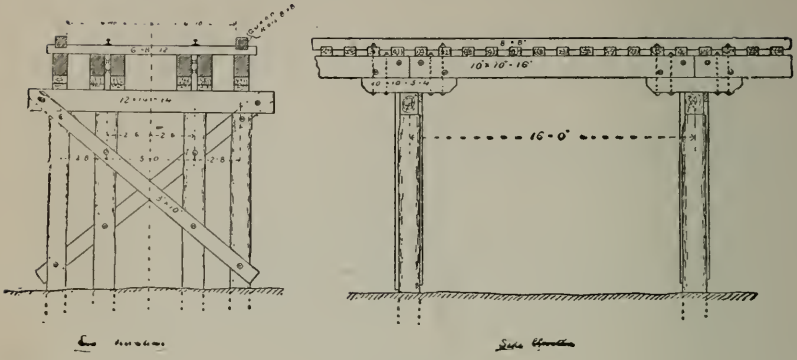
FIG. 166. PILE TRESTLE BRIDGE.
