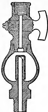
FIG. 28. SECTION OF SIPHON.
