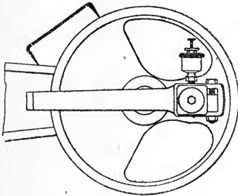
FIG. 23. TRAM ON DISC.
