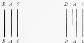
FIG. 1.—NORMAL TRIPLET.
