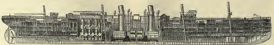
Longitudinal Section of the Champagne .
