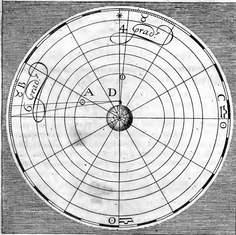
FIGURA PARALLAXEOS OBSERVATIONEM OSTÈDENS.
