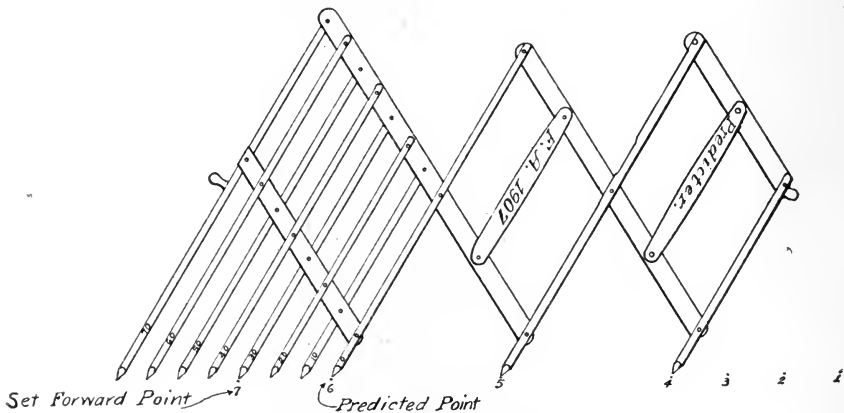
FIG. 49.—Mortar Predictor.
