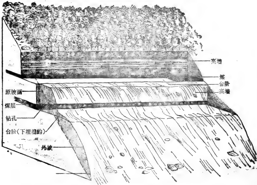
图8-12 该图示山坡上平面露天开采复合层的特征。虚线示原坡面，裸露在上方地层的是壁面、一些未开采的煤层和阶地。阶地一部分是由采煤后所遗留的坚硬岩床所组成，一部分是由覆盖层所组成，覆盖层从顶层被推到底层的阶地上，覆盖住阶地、壁和裸露的煤层。请注意在更低一层中的垂直孔穴，在覆盖层太厚以致无法把它们移走的地方采用钻孔机采煤，从而造成这些孔穴。从第一个挖方起覆盖就被推下山坡。覆盖层的不稳定性是由于被推下山坡的挖出的土石缺乏支撑基础，外坡的较低部分无法支撑住上面压下的重量，因而造成整个地层滑坡，结果产生山崩。
