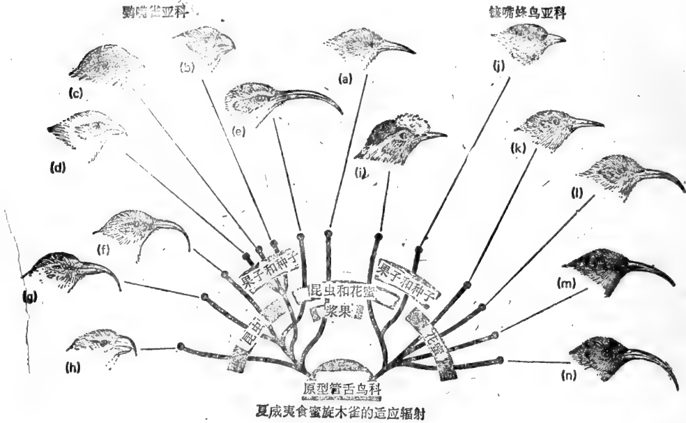
图2-15 夏威夷管舌鸟科食蜜旋木雀的适应辐射。所选出镰嘴蜂鸟 (Drepanidinae) 和鸚嘴雀 (Psittirostrinae) 两个亚科的代表表明这个科如何从一个普通的原始亲本通过适应辐射进化。两个亚科显示以食物为基础的一定程度的类似进化。(a) 绿管舌鸟 ( Loxops virens )，除以花蜜和浆果为食物外，还觅食树皮裂缝中和树叶包卷着的虫子。(b) 科纳鸚嘴雀 ( Psittirostra kona )，食种子鸟，已绝灭。(c) 鸣唱鸚嘴雀 ( P. cantans )，食物广泛，有种子、虫子、昆虫幼虫和果子等。(d) 鸚嘴雀 ( P. psittacea )，食种子鸟，特别是食一种攀援藤露兜树 ( Freycinetia arborea ) 的种子。(e) 短嘴导颚雀 ( H. lucidus )，食昆虫。(f) 短嘴导颚雀 ( H. lucidus )，食昆虫。(g) 导颚雀 ( H. wilsoni )，食昆虫。(h) 拟鸚嘴雀 ( Pseudonester xanthophrys )，食天然天牛科的幼虫、蛹以及甲虫，用弯曲的上喙勾挂树枝。(i) 冠施蜜鸟 ( Palmeria dolei )，食昆虫和光叶七叶树 (ohio) 的花蜜。(j) Cirridops ana ，食果子 and 种子，已绝灭。(k) 白臀蜜鸟 ( Himatione sanguinea )，食 Meirosideros 的花蜜和毛虫。(l) 鸚嘴管舌鸟 ( Vestiaria coccinae )；食各种花的蜜和圈毛虫 (loop caterpillars)。(m) 黑镰嘴蜂鸟 ( Drepanis funerea )，食花蜜，已绝种。(n) 太平洋镰嘴蜂鸟 ( Drepanis pacifica )，食花蜜，已绝种 [依 Amadon (1947, 1950) 和其他来源的资料绘制；进化资料引自 Amadon]
