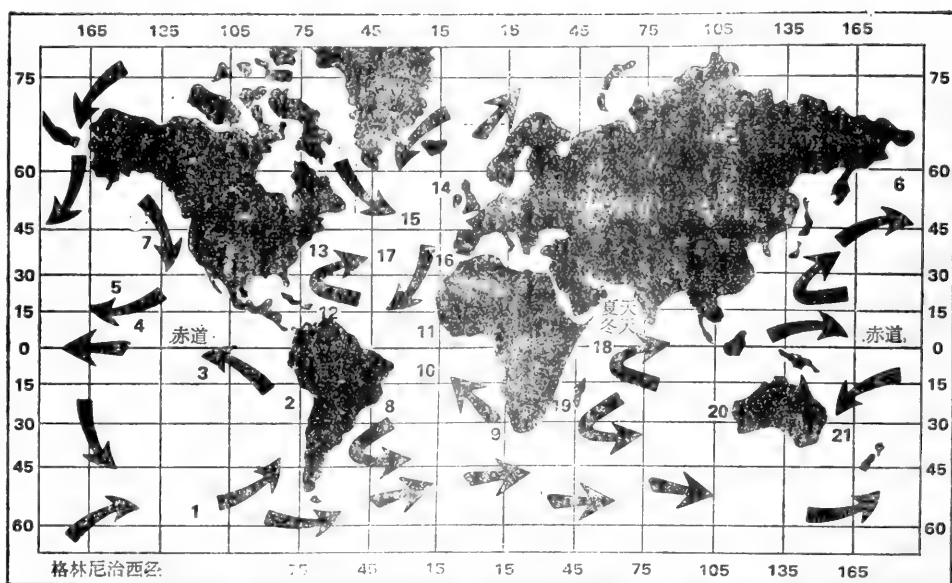
图14-3 世界的海流。注意海流的循环是如何受大陆地壳影响的，各个海洋是如何通过海流而互相联系的。(1) 南极西风漂流；(2) 秘鲁海流，或叫亨伯特海流；(3) 南赤道流；(4) 赤道逆流；(5) 北赤道流；(6) 黑潮；(7) 加利福尼亚海流；(8) 巴西海流；(9) 本格拉海流；(10) 南赤道流；(11) 几内亚海流；(12) 北赤道流；(13) 墨西哥湾流；(14) 挪威海流；(15) 北大西洋海流；(16) 加那利漂流；(17) 马尼藻海；(18) 季风漂流(夏天自东方来，冬天从西方来)；(19) 莫桑比克海流；(20) 西澳大利亚海流；(21) 东澳大利亚海流(引自Coker, 1947)
