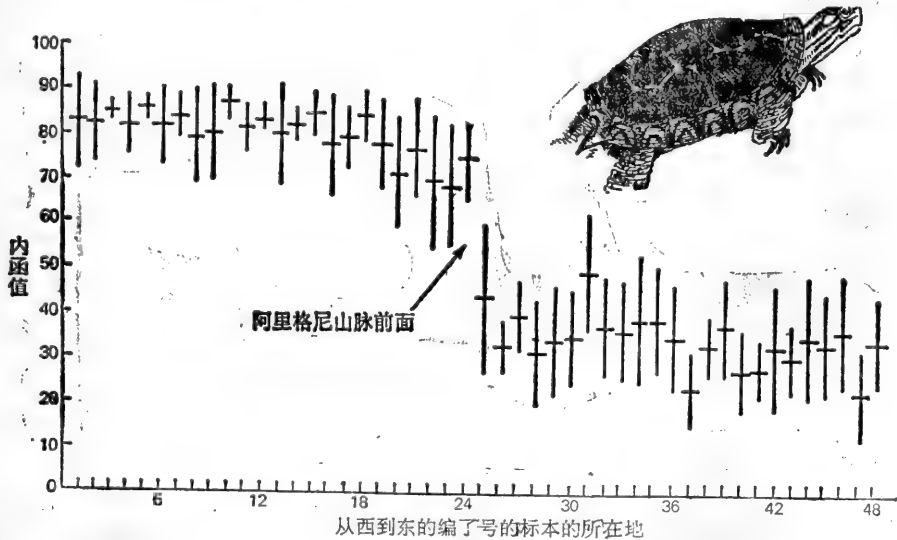
图 2-13 锦龟 ( Chrysemys picta ) 由两个亚种组成: 东部锦龟 ( C. P. picta ) 和中部锦龟 ( C. p. marginata )。在阿巴拉契亚高原的北部, 两个亚种间渡。在西弗吉尼亚, 阿巴拉契亚高原构成一道生态的、地理的屏障, 有效地把两个亚种隔开。这种隔离用诸如缝线排列、背甲的宽度和图案等等一些可测量的特征的综合值的区别图说明。竖条是平均值, 横条是标准差 [引自 L. Clack (1975) 未发表资料]
