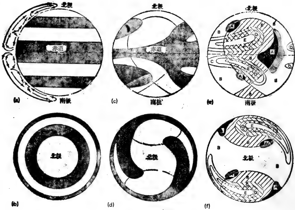
(e) 和 (f) 部分中的字母和暗影代表地球的气候条件，下列为Thorntwaite's 的分类系统：
