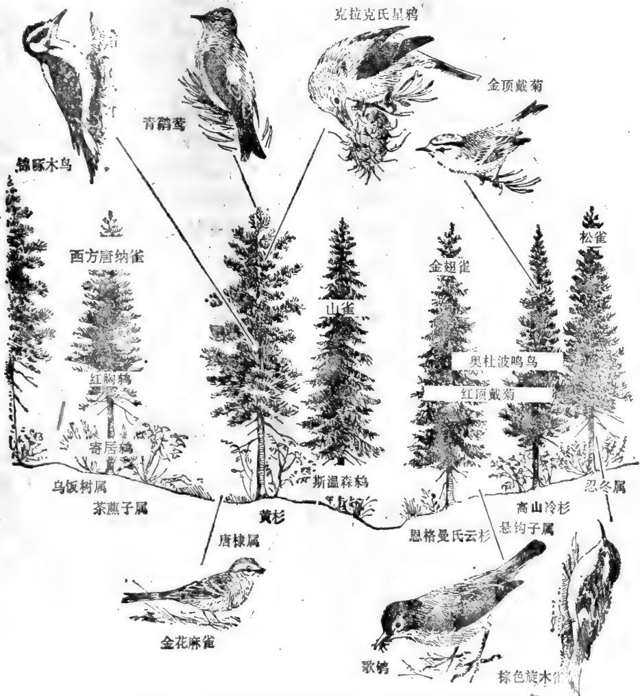
图23-8 在怀俄明州的云杉-冷杉林中某些鸟类的取食生态位
