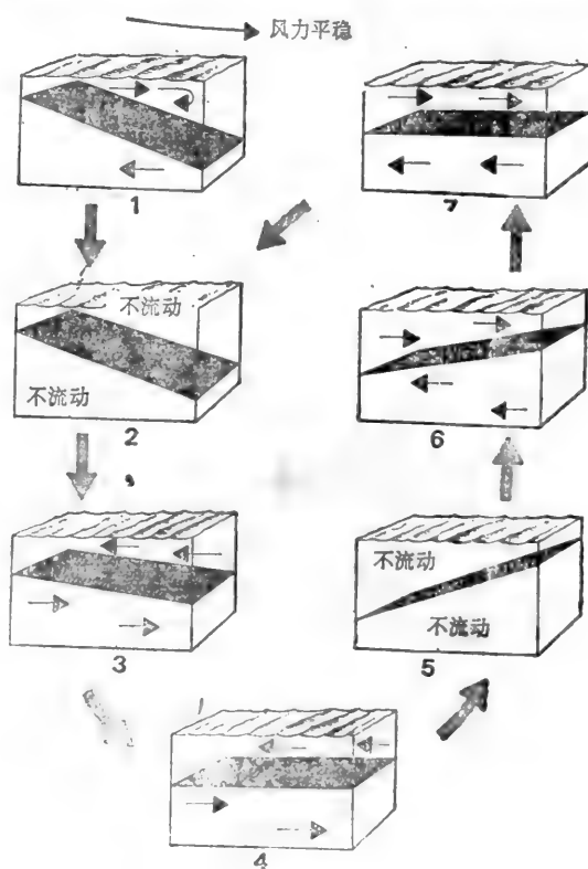
图11-2 温跃层斜坡和风停息后发生的静振的图解说明
