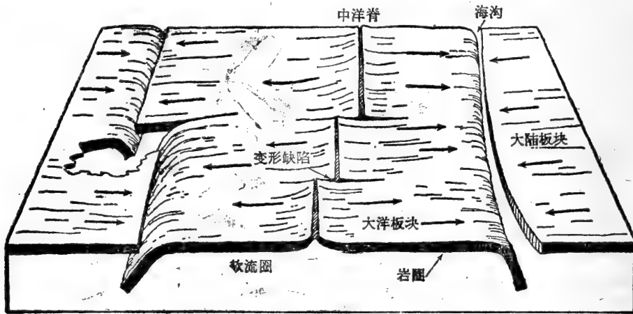
图2-1 根据全球构造理论的板块学说,地球的外壳(洋壳和陆壳)系由漂浮在已经变形的、无强度的软流圈上的一小块块板状坚实脆性岩圈组成。全球有六大坚实板块, 其中的每一块都象水一样移动, 而且, 当它们掠过软流圈时, 甚至可能旋转。这些板块可分开移动, 这时加宽板块间的缝隙; 它们亦可一起移动, 这时使地壳沿板块破裂; 它们还可滑过另一板块。在洋底下面分开的板块产生中洋脊; 板块会合处, 一板块的一端向下弯曲挤进软流圈(引自A. N. Strahler, 1971)
