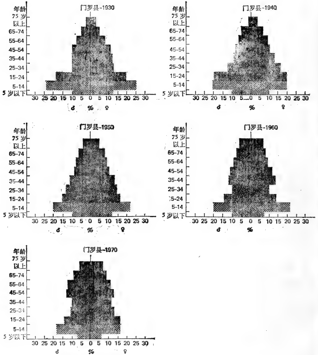
图9-20 西弗吉尼亚南方的门罗县1930—1970年间农业人口年龄金字塔，因为在美国统计方法易变，人口调查署细分了在不同的人口调查期县人口的龄级，除了0—5岁龄级以外，龄级的划分是10年年龄组代替了5年年龄组，保留0—5岁的年龄组是为了表示出生率缓慢的变化，详见文内的描述（R.L.Smith绘制的金字塔是引用美国人口调查署的资料，引自R.L.Smith, The Ecology of Man, An Ecosystem Approach , Harper & Row, New York, 1976）
