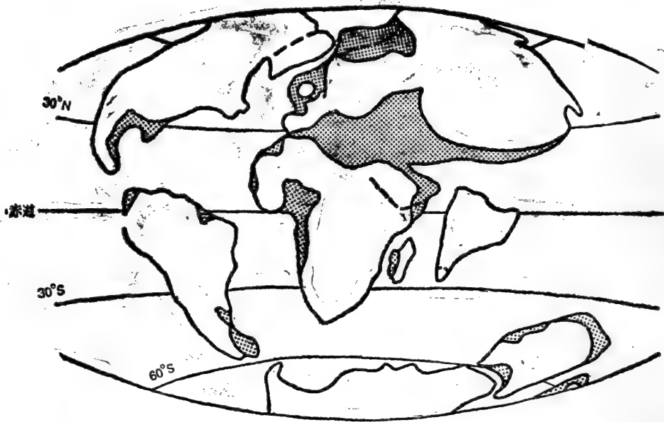
图2-5 5千万年前的下第三纪(上始新世)时的地球。虚线表示现在的海岸线。阴影区表示浅陆缘海。这时期,北美与欧洲大陆已分开,南美与非洲完全分开了,澳大利亚与南极洲已分开(引自Cox等,1973)。
