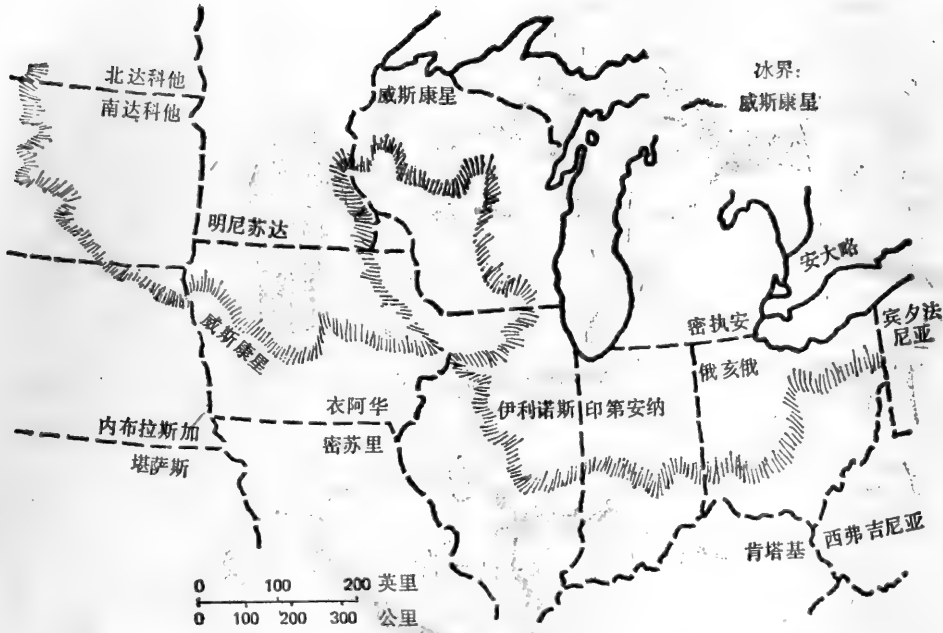
图2-6 更新世时，北美洲北部被四块冰川覆盖。每一冰川的边界常以尾迹标明。最后的，而且也许是最有意义的冰川是威斯康星冰川，如线标明 (引自A.N. Strahler, 1971)
