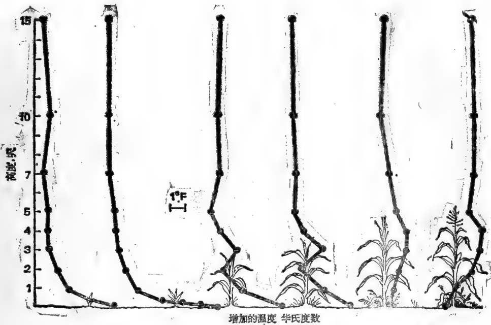
图6-20 玉米地从幼苗到收获, 正午的垂直温度梯度。注意作用面高度的增加 (引自Wolfe等, 1949)
