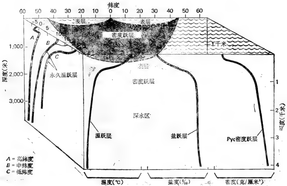
图14-1 海水温度和盐度的综合断面图。左侧面以一般方法说明海洋的温度断面。(A) 北极地区或高纬度地区。注意：低盐度的较冷表层水是在较暖、含盐量较高的水层上面。(B) 在中纬度，海水有季节性变化的表层温度和永久温跃层。(C) 低纬度的海水具有稳定的表层温度和永久温跃层 [引自 R.V. Tait, 1968, Elements of Marine Ecology (海洋生态学原理), Plenum, New York]。
