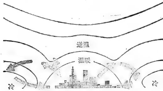
图6-24 晴朗无风天气，城市上空夜间循环的理想图。城市上空形成一个热岛。同时，乡村形成地面大气逆温。由此导致冷空气流向城市，城市夜间出现乡村微风。曲线表示温度等温线；箭头代表微风（引自H. Landsberg, 1970, science, 170:1271）
