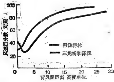
图6-21 背风面稀疏桦林, 三角叶杨和洋槐林地上16英寸处的风速比较。桦的曲线说明稀疏林分的有效性, 风可以在树冠下流动。障碍物背面是起点 (引自Stoockeler, 1962)
