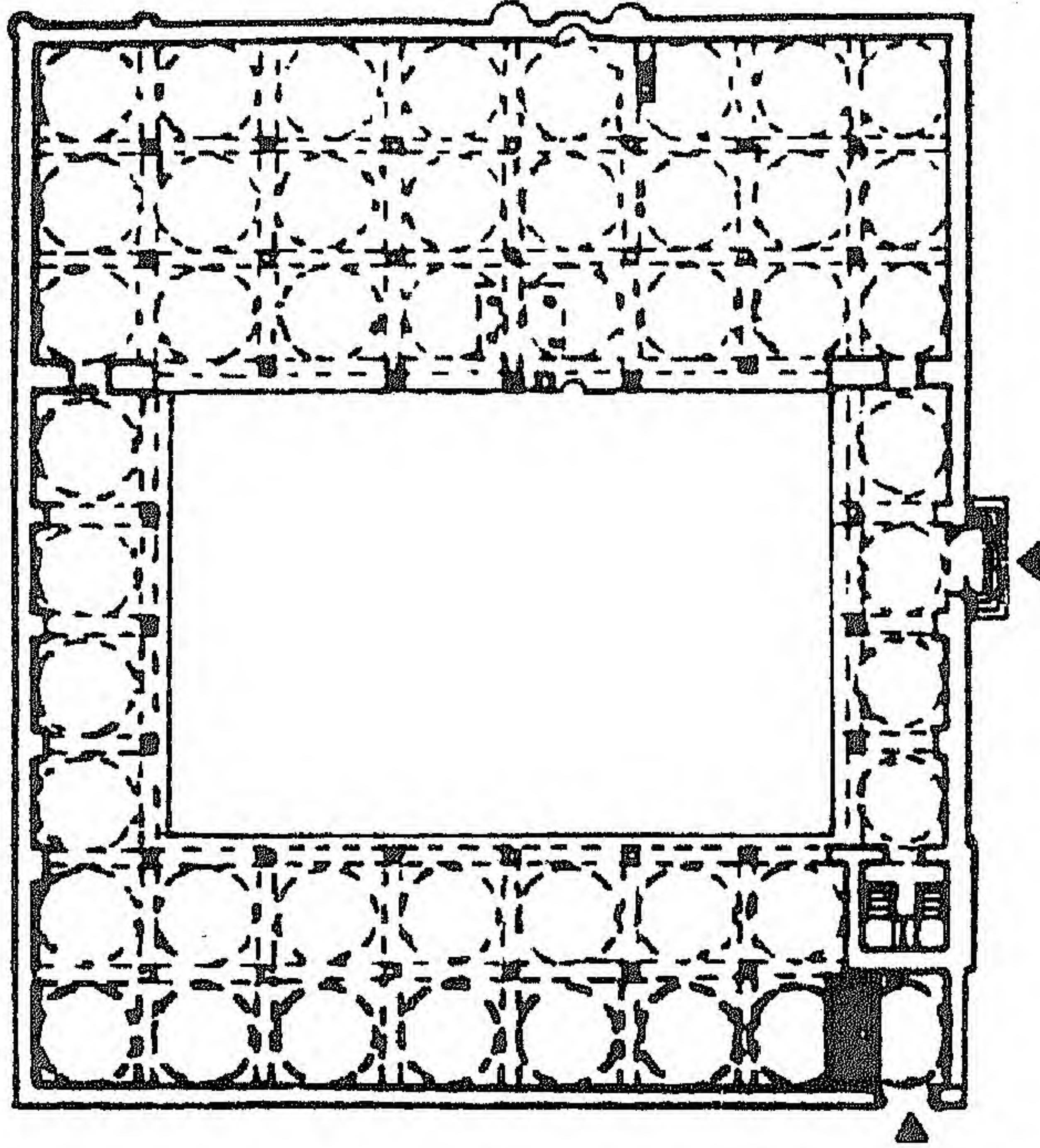
شكل ( ٥ ) : مسقط أفقى لمسجد قباء .
