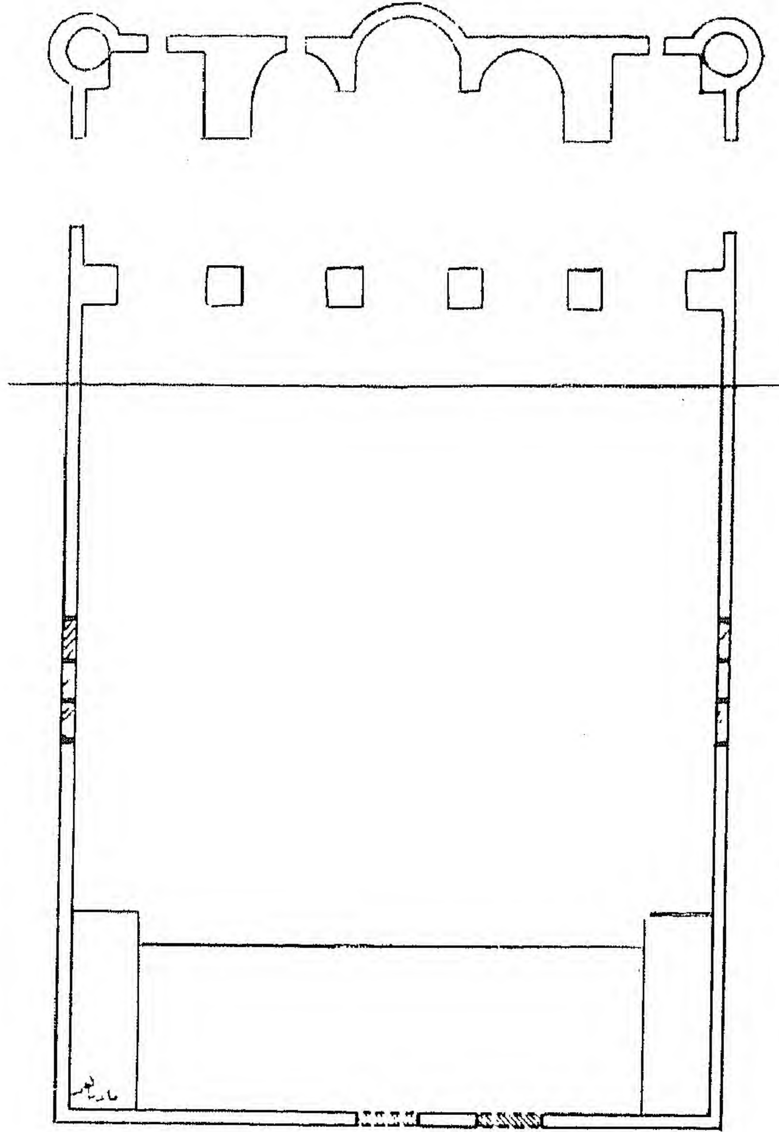
شكل رقم (١) تخطيط مسجد البيعة الكبرى .
