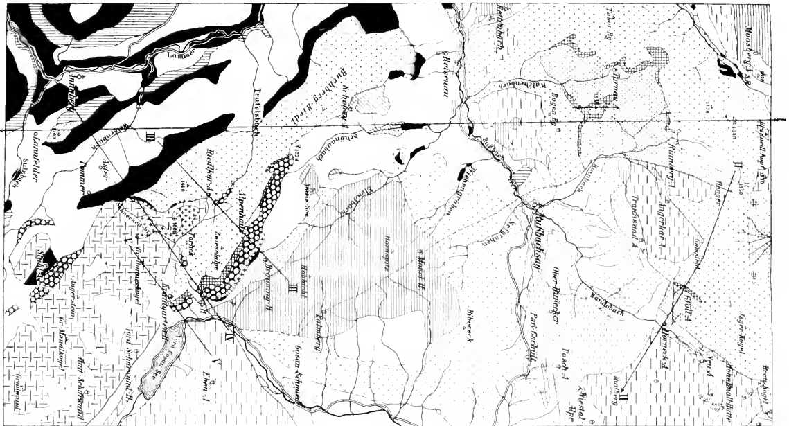
Geologische Karte des Beckens von Gosau.
