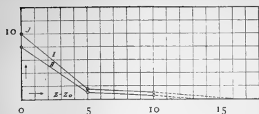
Kurve 7. Entladungspotential 21800 Volt. Blättchendicke = 1.90 \mu .
