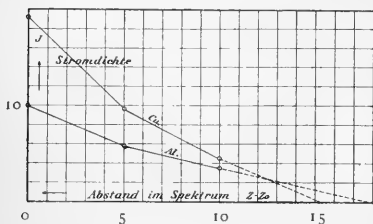
Kurve 1. Entladungspotential = 16500 Volt.
