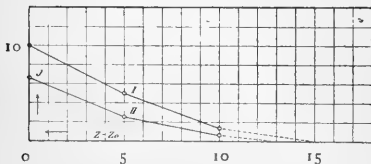
Kurve 3. Entladungspotential 16500 Volt. Blättchendicke = 0.53 \mu .
