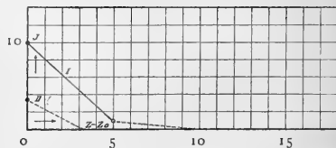
Kurve 5. Entladungspotential 27800 Volt. Blättchendicke = 0.53 \mu .
