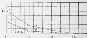
Kurve 4. Entladungspotential 21800 Volt. Blättchendicke = 0.53 \mu .
