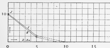
Kurve 9. Entladungspotential 27800 Volt. Blättchendicke = 2.55 \mu .
