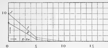
Kurve 8. Entladungspotential 21800 Volt. Blättchendicke = 2.55 \mu .
