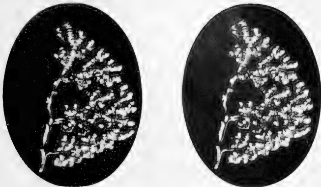
Fig. 1. Photostereogramm des Metallausgusses von Bronchuli mit Alveolarbäumchen der Lunge von Mus rattus L. Vergr.: \frac{10}{1} .
