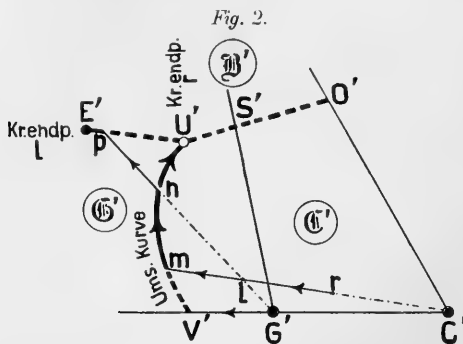
Charakteristische Verschiedenheit der Kristallisationsbahnen rmU' und lmnpE' .
