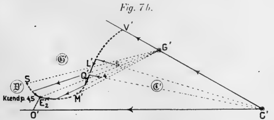
Strukturfelder und Kristallisationsbahnen in der Projektion \mathcal{C}' der Sättigungsfläche der Komponente C = NaCl .
