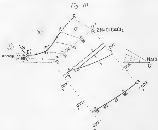
Kristallisationsbahnen der Lösungen des Schnittes IX mit dem zugehörigen Konzentrations-Temperatur-Diagramm.
