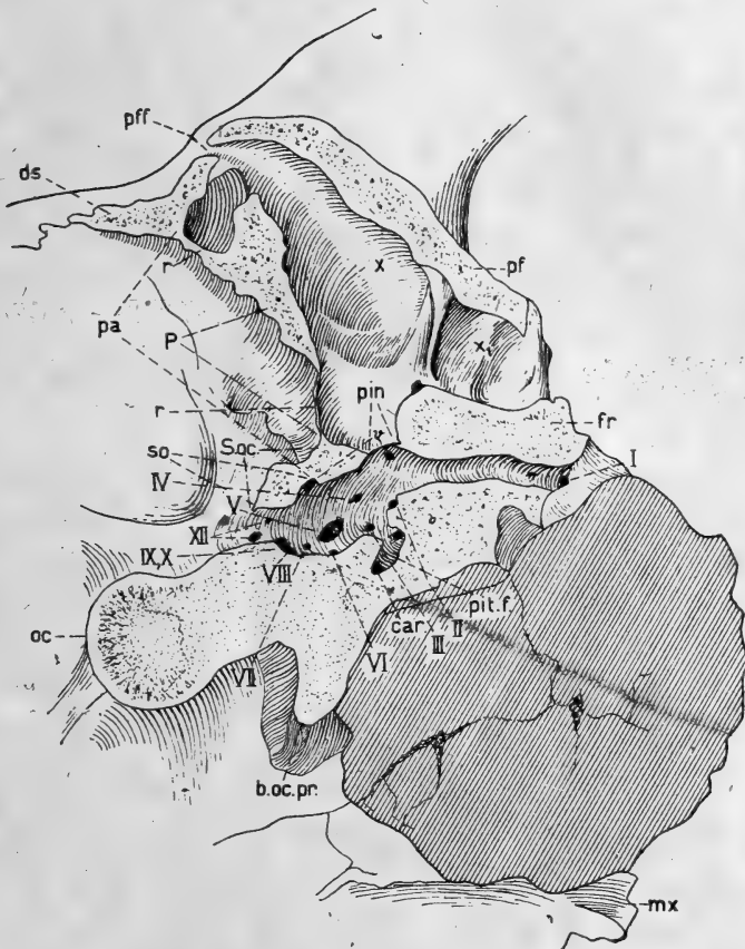
Fig. 1. Triceratops sp. Oberste Kreide; Doegie Creek, Niobrara County, Wyoming. Längsschnitt durch den Hirnschädel in etwa \frac{1}{8} nat. Gr. aus GILMORE 1919, S. 103, Fig. 1 und Taf. 8. (Die durchschnittenen Knochen sind punktiert, die Bezeichnungen z. T. geändert).
