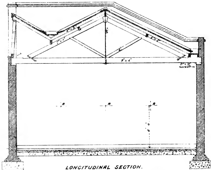
LONGITUDINAL SECTION.
