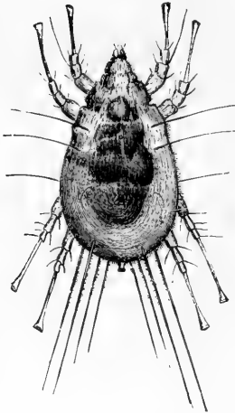
FIG. 919.— Sarcoptes Hippopodus .
