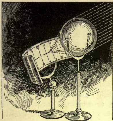
Fig. 3.—A Tell-tale for the Sun.
