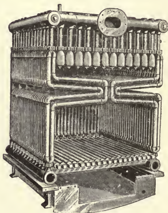
FIG. 90.—ALMY, 1890.
