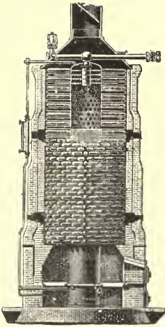
FIG. 77.—HAZELTON, 1883.
