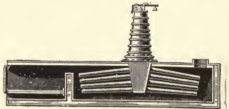
FIG. 69.—JOHN STEVENS, 1803.
