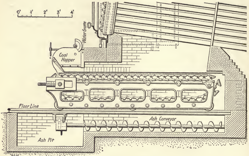
Longitudinal Section.
