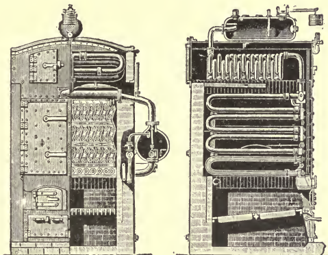
FIG. 85.—BELLEVILLE, 1865.
