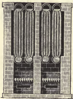
FIG. 81.—ROWAN, 1865.
