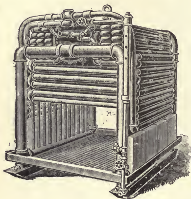
FIG. 89.—ROBERTS, 1887.
