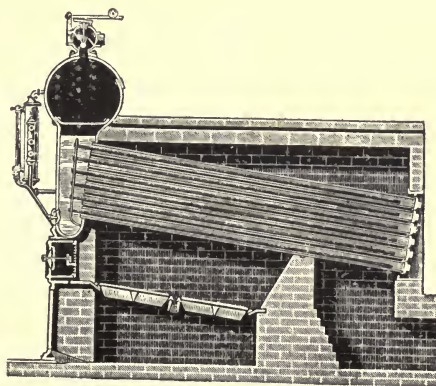
FIG. 73.—MILLER, 1870.
