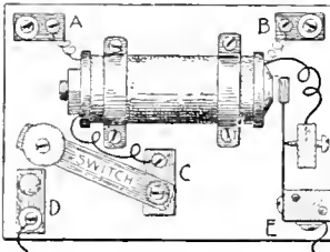
FIG. 24. AN INTERRUPTER.
