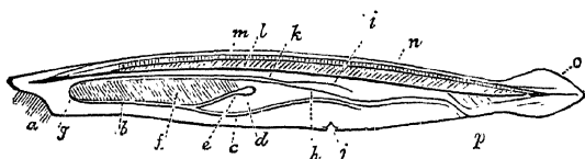
FIG. 56—Lancelet.
