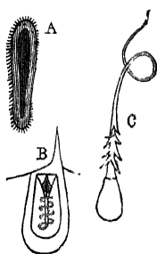
FIG. 39.—Hydra.
