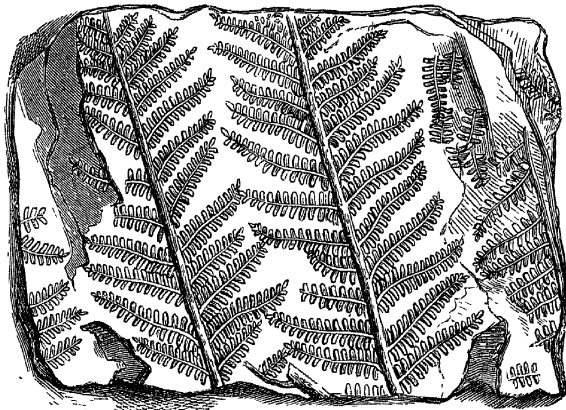
Tree Fern.
