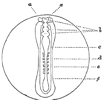
FIG. 69.—Embryo Stage.
