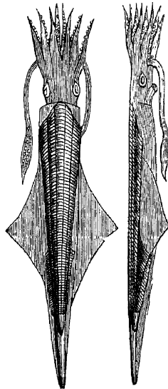
FIG. 14 —Belemnites.
