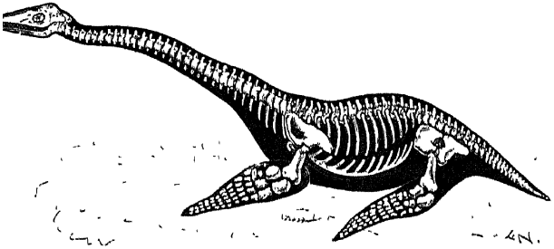
FIG. 15.—Plesiosaurus.
