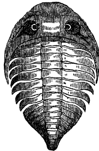
FIG. 10.—Trilobite.
