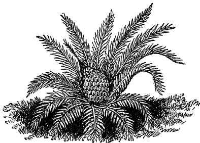
FIG. 32 —Cycad (Australia).
