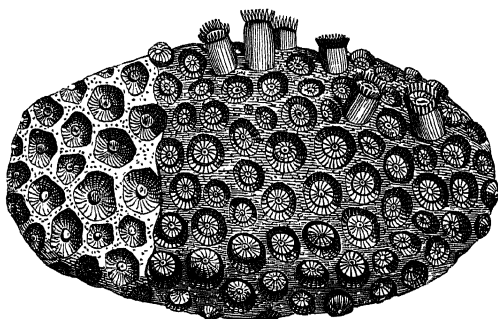
FIG. 42.—Coral.
