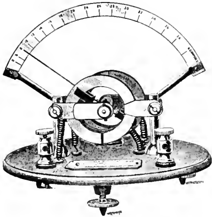
I H A. C. AND D. C. AMMETER.
