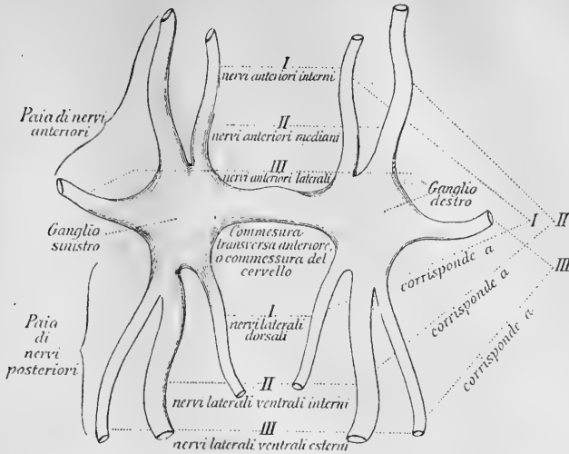
Fig. 2. Schema del sistema nervoso dei Distomidi (dal dorso).
