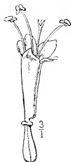
Fig. 301. Valeriana sambucifolia.
