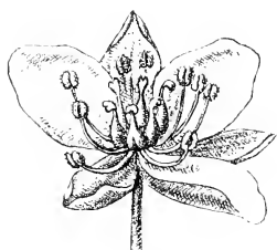
Fig. 23. Butomus umbellatus .
