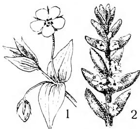
Fig. 253. 1 Anagallis , 2 Glaux .
