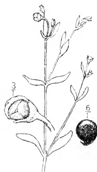
Fig. 155. Montia lamprosperma .
