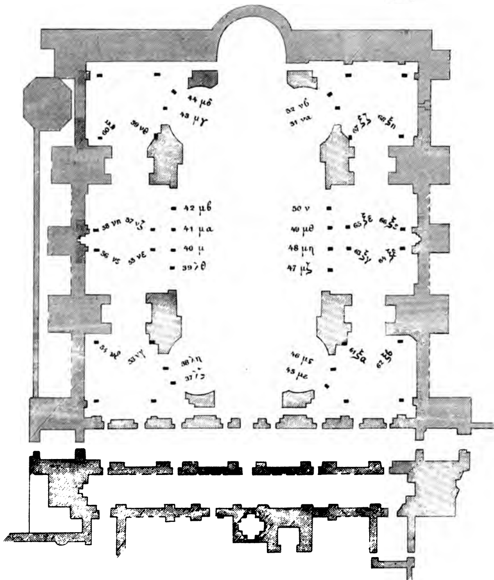
Τὸ σχέδιον τοῦ Ναοῦ τῆς Ἁγίας Σοφίας.
