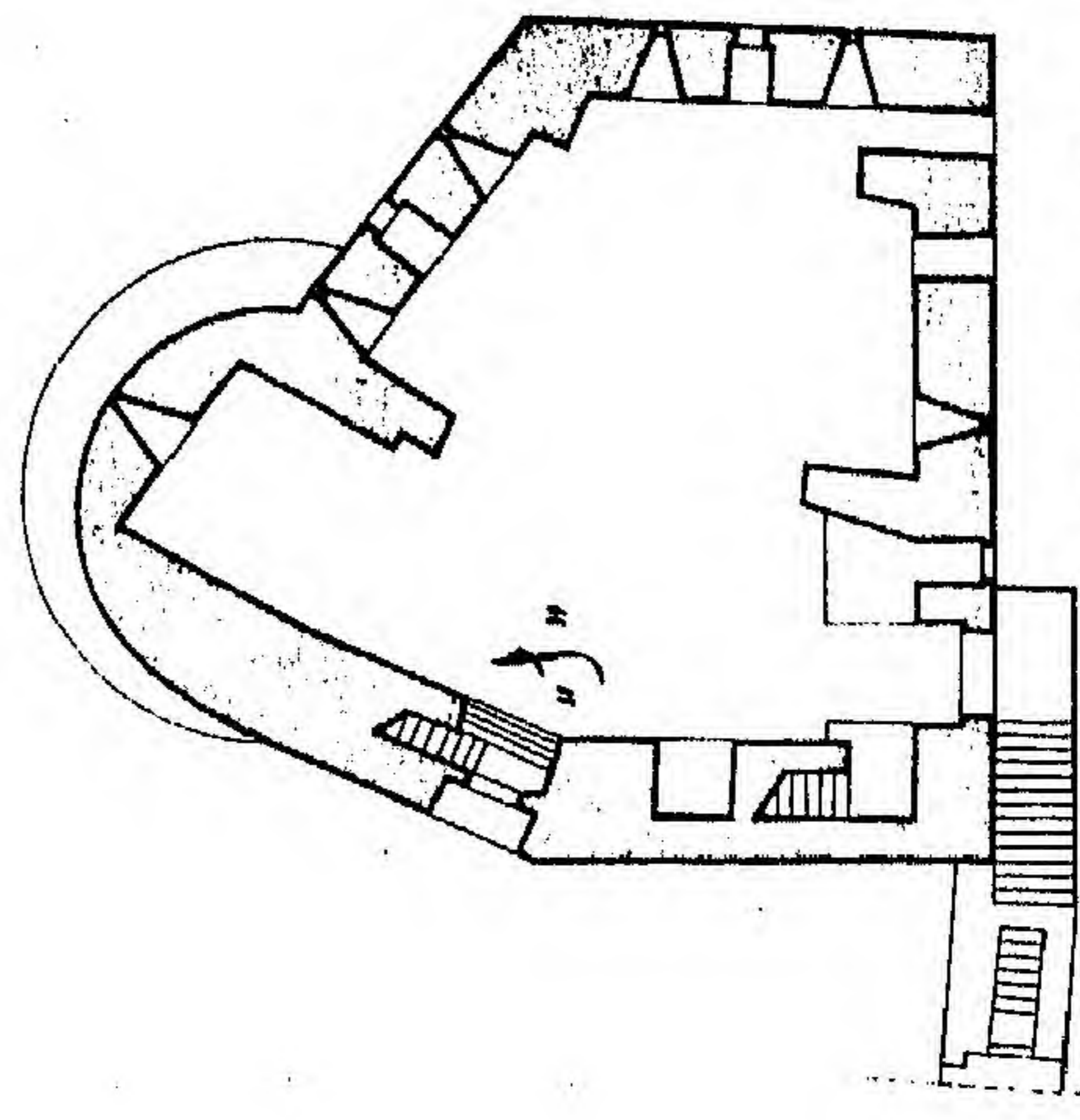
تخطيط للبيج المملوكي مقياس ١/٤٠٠
