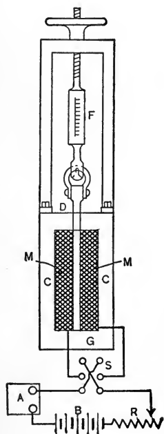
Fig. 9A. Thompson Permeameter.
