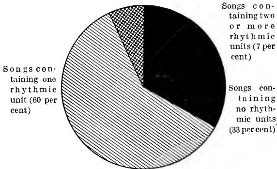
FIG. 17. Rhythmic unit.
