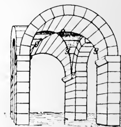
FIG. 47.—GROINED VAULT. g. g. Groins.
