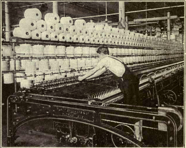
FIG. 24.—MULE SPINNING.
