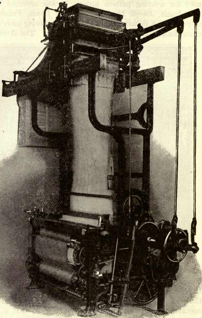
FIG. 27. — JACQUARD LOOM.
