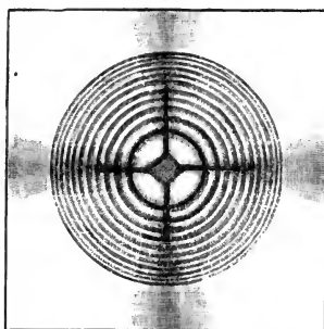
Fig. 182.—( \alpha - \beta = 90^\circ ).
