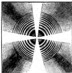
Fig. 181.—( \alpha - \beta = 0^\circ ).
