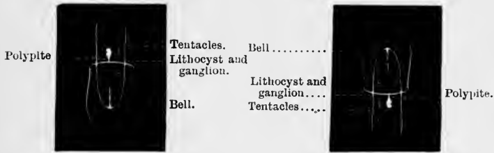
FIG. 28. Medusa (Sarsia), natural size.
