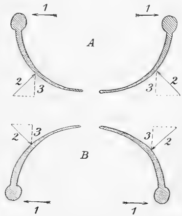
Abb. 120. Schema der Kraftwirkung an der heterozerten Schwanzflosse. A bei ventraler und B bei dorsaler Flossen-zahne. Der Pfeil 1 zeigt die Bewegung der Flossenachse, Pfeil 2 die Richtung des Wasserwiderstandes senkrecht zur Zahne, der sich in zwei Komponenten, eine horizontale, von der Achsenbewegung überwindene, und eine vertical (3) nach oben (A) bzw. unten (B) wirkende zerlegen läßt.
