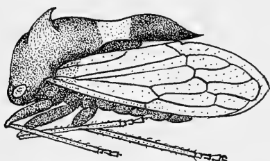
Fig. 4. Tricentrus carinatus sp. nov.
