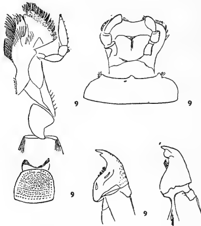
Fig. 9. Tetralanguria splendens .
