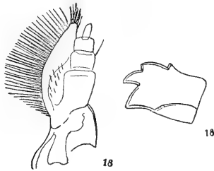
Fig. 18. Eutrachelus Temmincki .
