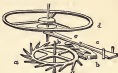
Lever Escapement.
