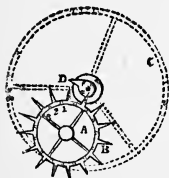
Duplex Escapement.
