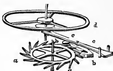
Lever Escapement.
