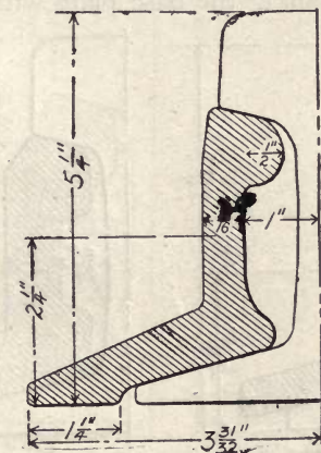
Section of C. R. R. of N. J. Rail Joint.
