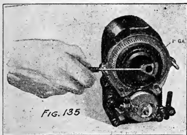
Fig. 135. Testing magneto.
