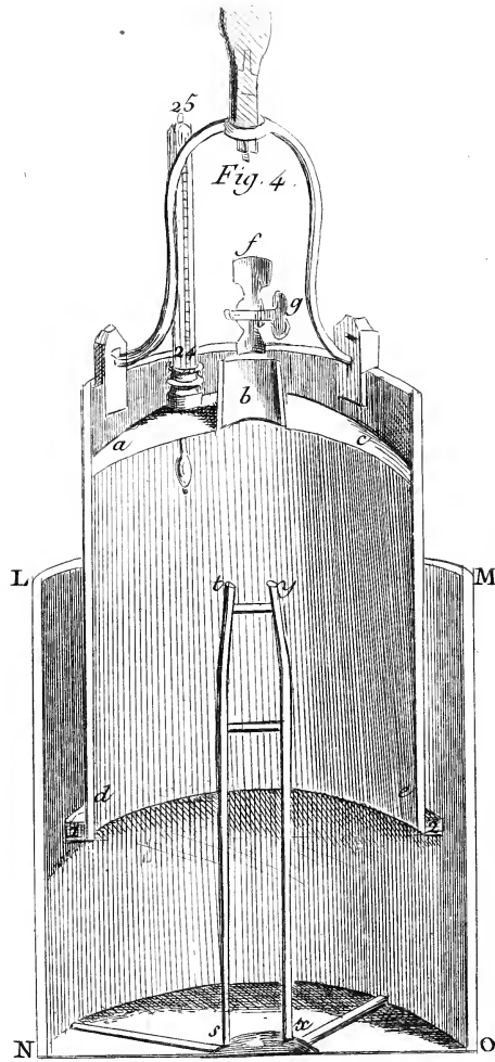
Echelle de 5 Pieds .
