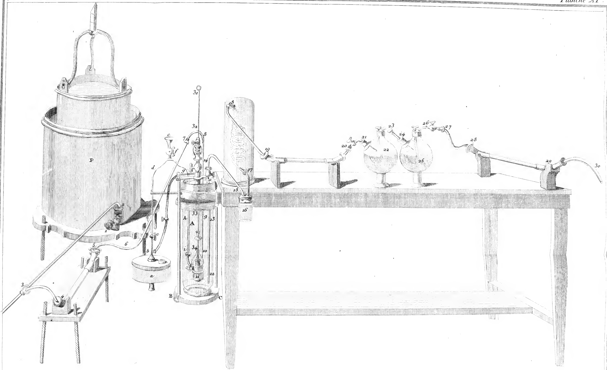
Echelle de 4 Pieds
