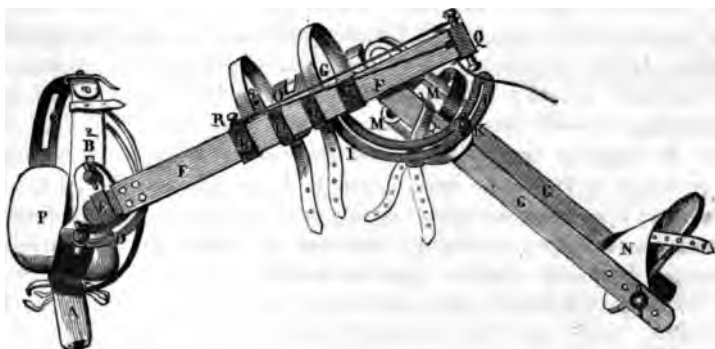
FIG. 173. — Appareil de Ferd. Martin. — Partie de l'extension et de la contre-extension montées.
