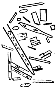
FIG. 48. — Urée. (Beale.)
