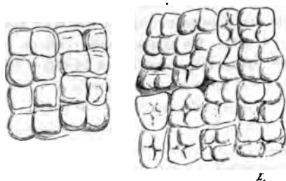
FIG. 1. — Sarcine.
