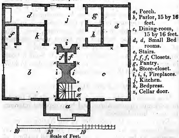
Ground-plan.
