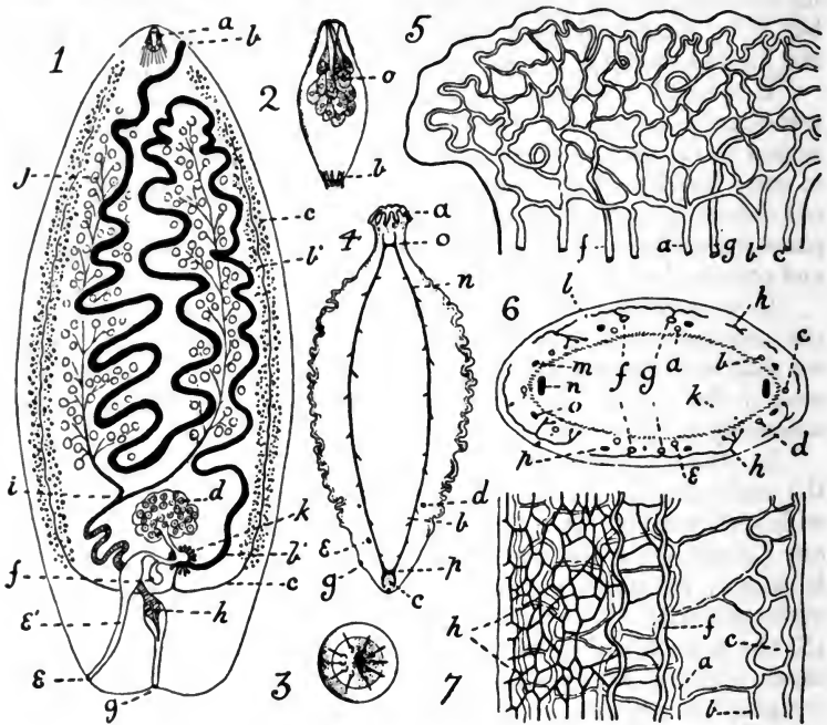
FIG. II.—Monozoa.
