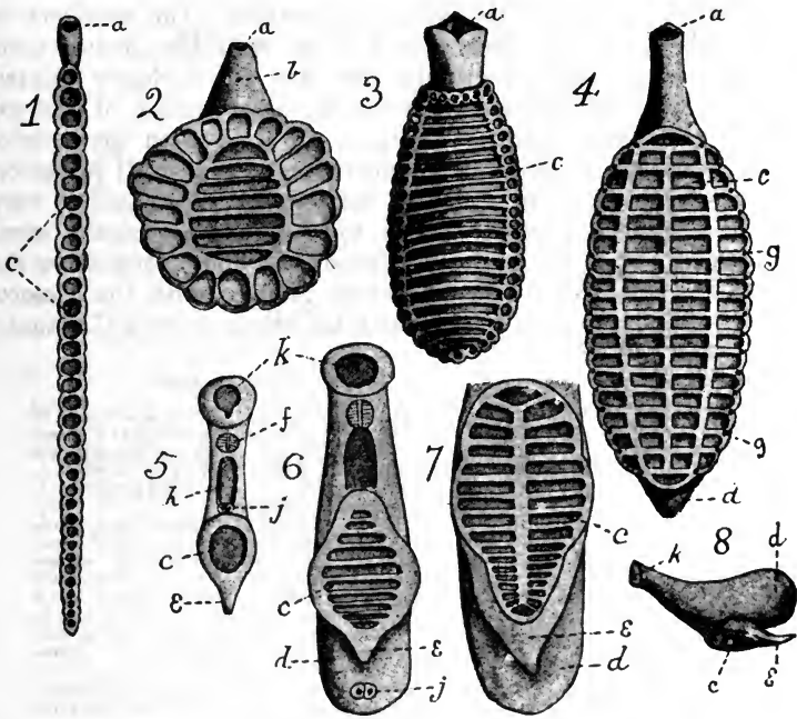
FIG. VI.—Aspidocotylea.
