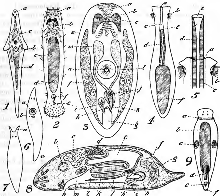
FIG. III.—Rhabdocoelida.
