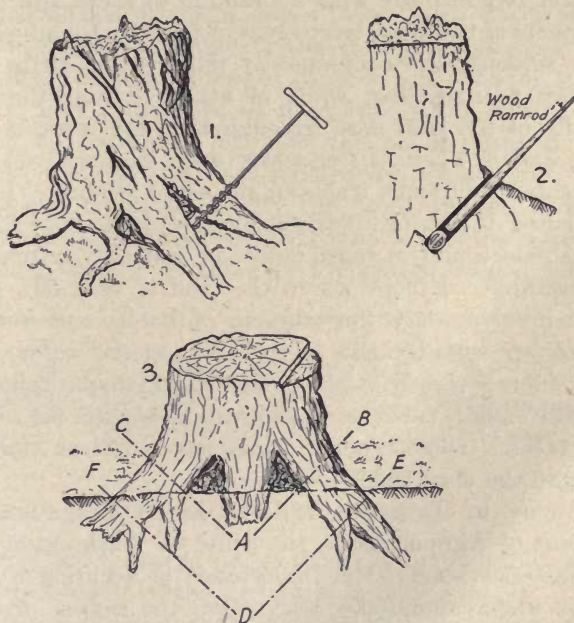
FIG. 24.—Blasting stumps.
