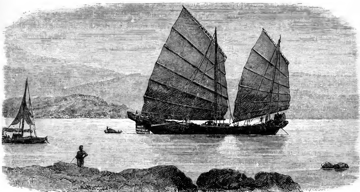
CHINESE JUNK.
